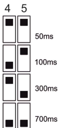
Рисунок 2.12 - Положение переключателей времени прерывания
