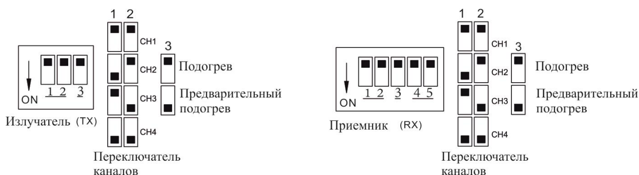
Рисунок 2.11 - Переключатель каналов
