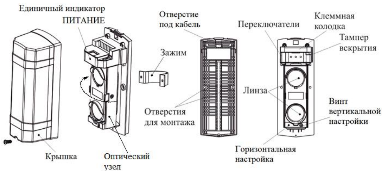
Рисунок 1.4 - Общий вид излучателя
