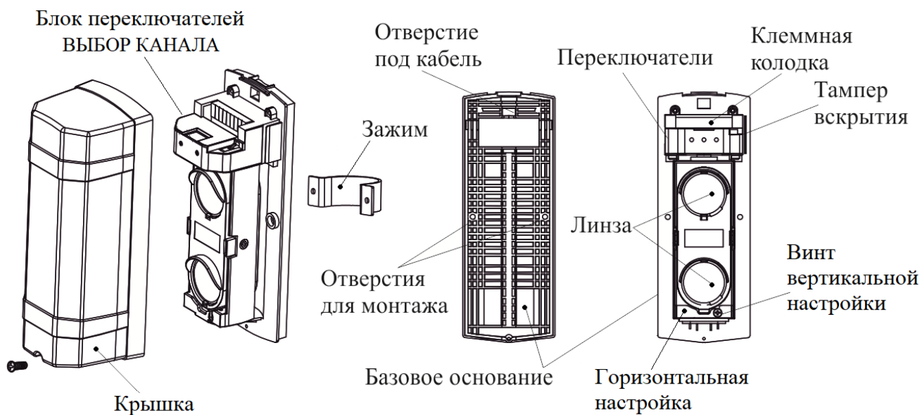
а) общий вид приемника
