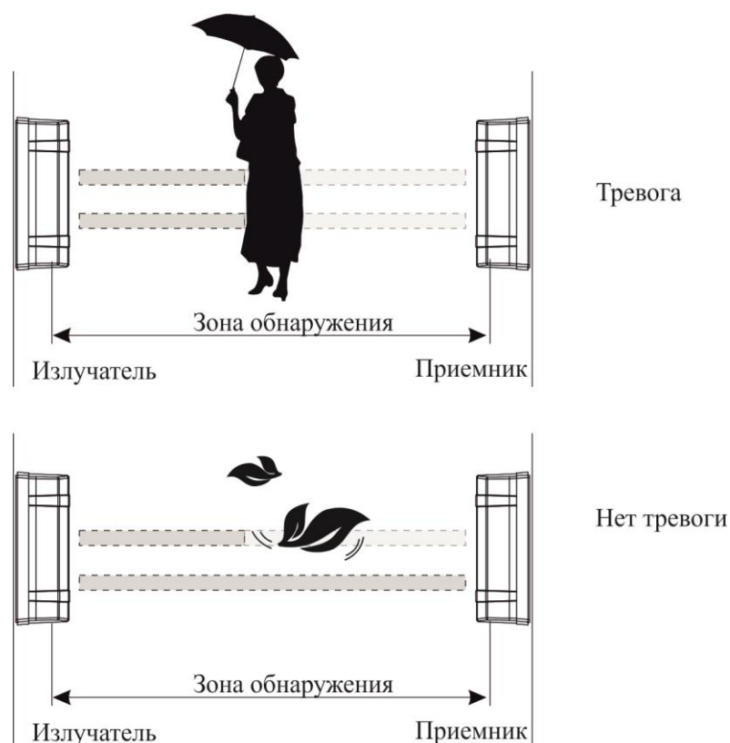
Рисунок 1.3 - Принцип действия извещателя
