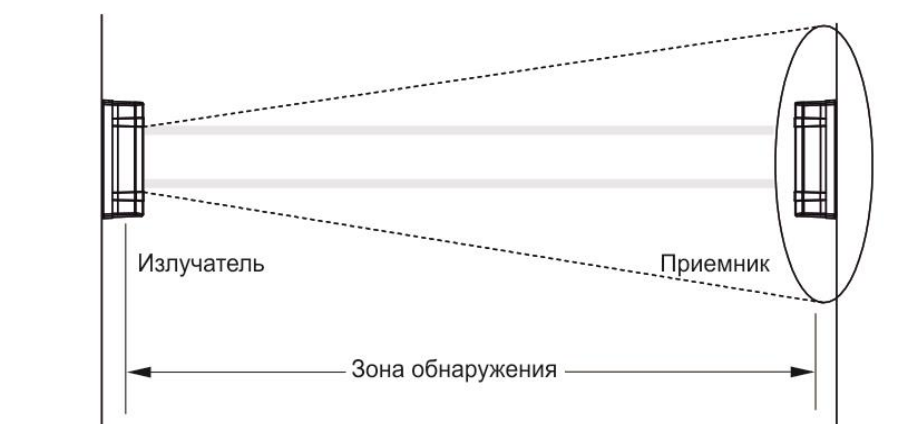
Рисунок 1.2 - Расположение БИ и БП при формировании ИК барьера
