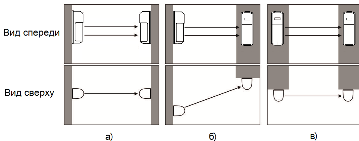
Рисунок 2.7 - Варианты расположения извещателей под разными углами
